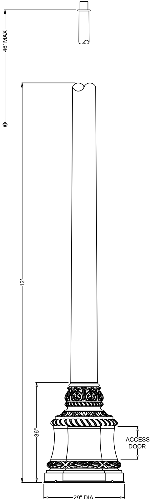
SMOOTH SHAFT N.T.S
